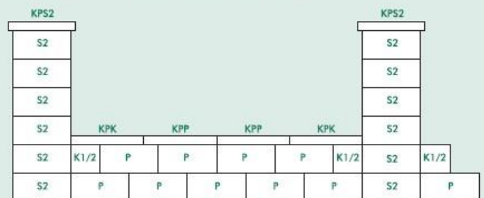
Príklad skladby plotu so stĺpovými tvárniciami S2
