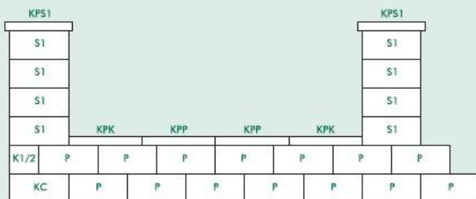
Príklad skladby plotu so stĺpovými tvárniciami S1
